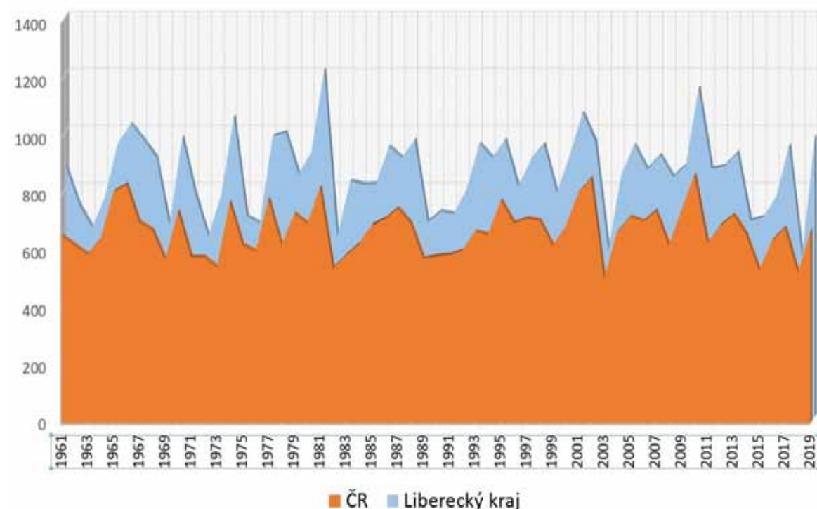
Úhrny srážek pro ČR a Liberecký kraj 1961 - 2019
